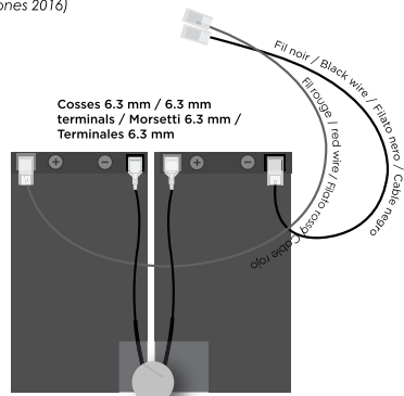
Branchement 24V sur séries ACCESS et OPEN versions antérieures à 2016 24V connection ( ACCESS and OPEN prior versions to 2016) Cablaggio 24V ( ACCESS e OPEN versioni precedenti a 2016) Cableado 24V ( ACCESS y OPEN versiones anteriores a 2016)
