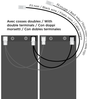
Branchement 12V sur versions antérieures à 2016 12 Volts connection prior versions to 2016 Cablaggio 12V versioni precedenti a 2016 Cableado 12V versiones anteriores a 2016
